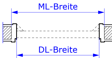
Schnitt CD
