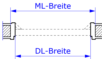
Schnitt CD
