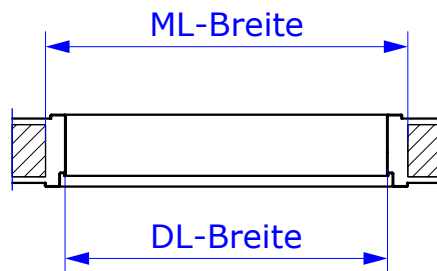
Schnitt CD
